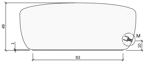
SECCIÓN A-A' / SECTION A-A'
