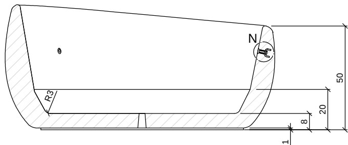
SECCIÓN A-A' / SECTION A-A'
