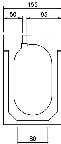
Ansicht A
