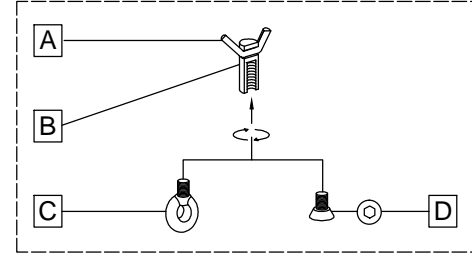
SISTEMA DE ELEVACIÓN / LIFTING SYSTEM
