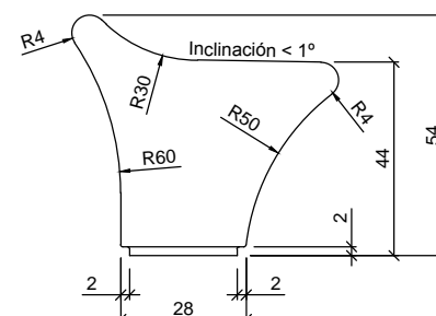
PERFIL / PROFIL VIEW
